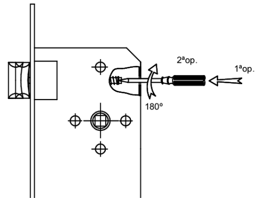
Reversibilidad picaporte. Latch reversibility
